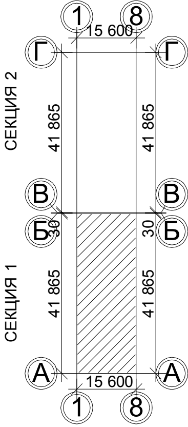
Компоновочная схема
